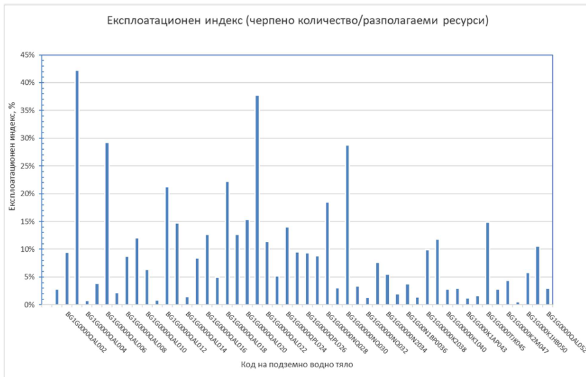
Фигура 2.1.4-3. Резултати за водния баланс на ПВТ – експлоатационен индекс. (източник БД)
