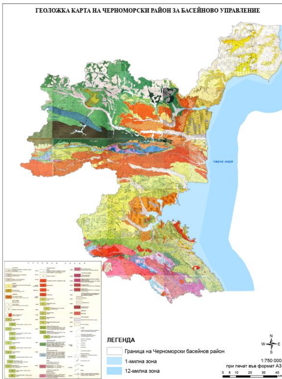
Фигура 2.1.4-13. Геоложка карта на Черноморски район за басейново управление. (източник БД)
