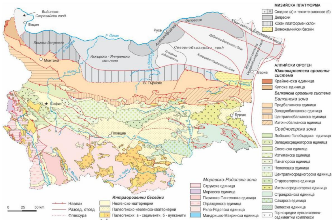
Фигура 2.1.5-2. Тектонска карта на България.
