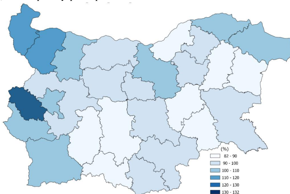
Фигура 2.1.1-5. Отклонения на годишния валеж през 2023 г. (%) спрямо климатичните норми през периода 1991-2020 г. (източник НИМХ)
