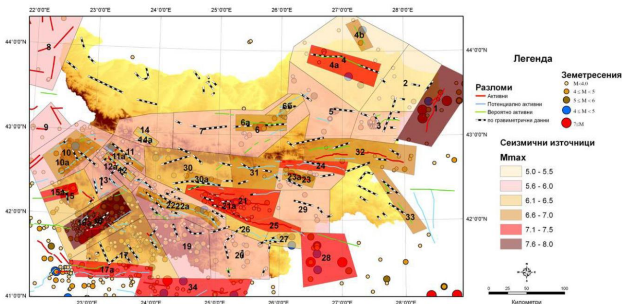
Фигура 2.1.5-6. Карта на сеизмичните източници. Източник: НИГГГ-БАН
