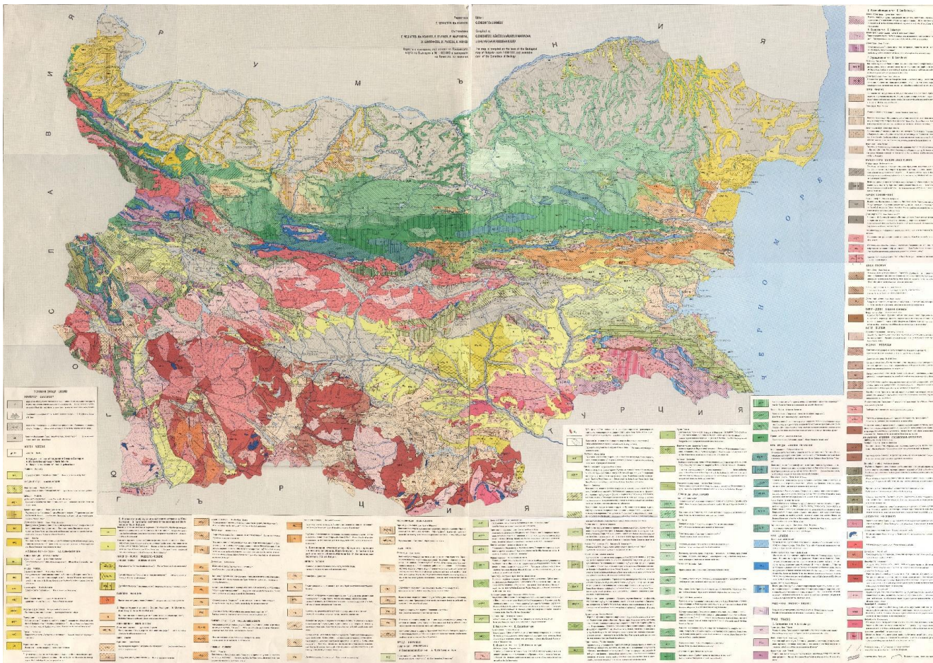
Фигура 2.1.5-1. Геоложка карта на България Източник: https://www.geokniga.org/
