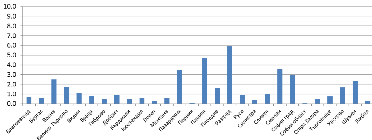
Фигура 2.1.11-3. Максимално измерени стойности в чувствителни райони в административните области на Р България (Обобщен доклад за електромагнитните полета в населените места в Република България за 2022 г., МЗ)
