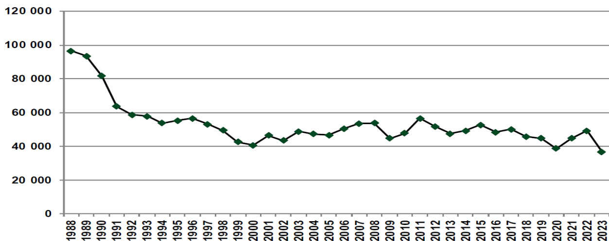
Фигура 2.1.1-11 Общи количества емисии на ПГ със сектор ЗПЗГС за периода 1988-2020 г., Gg CO 2 -екв. (източник UNFCCC)
