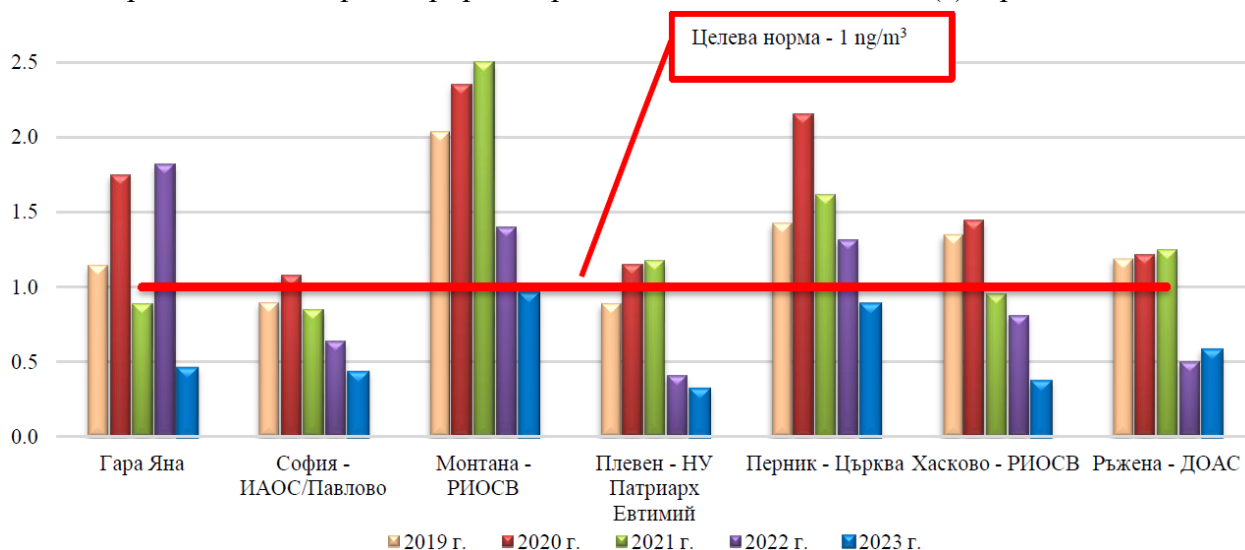
Фигура 2.1.2-9 Пунктове с превишение на СГН на бензо(а)пирен за периода 2019-2023 г., \text{ng/m}^3 (източник Национални доклади, ИАОС)
