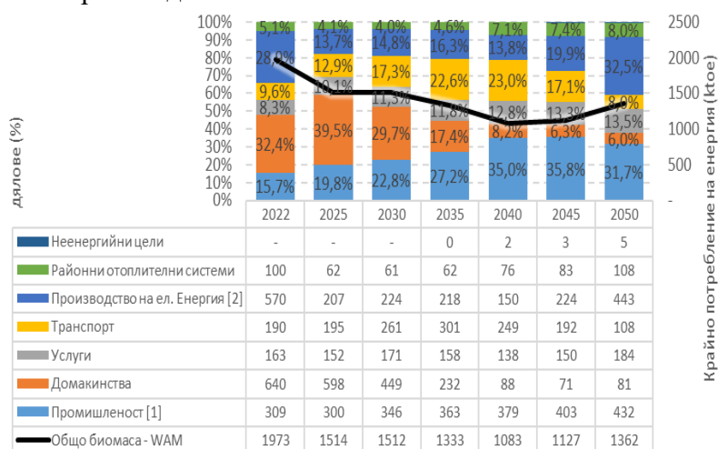
Фигура 1.2.1.1-5. Крайно потребление на твърда биомаса, биогаз и отпадъци по сектори (2025-2050 г.), ktce и дялове в % (източник – ИПЕК)
