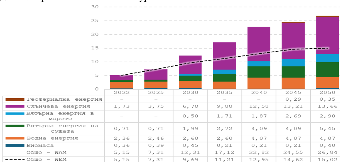
Фигура 1.2.1.1-2. Прогноза за инсталираните мощности за производство на електрическа енергия от ВЕИ по видове централи, GW (източник – ИПЕК)
