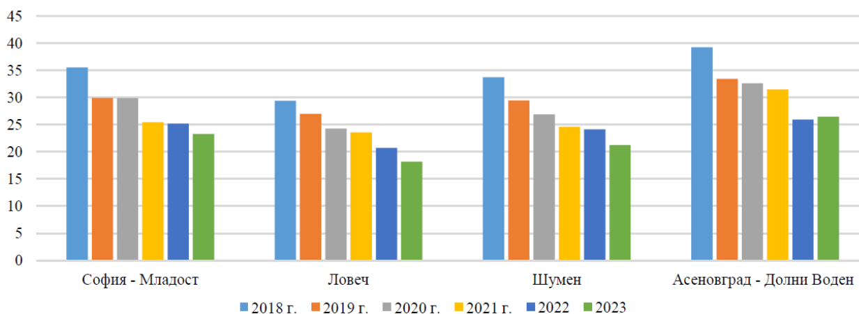
Фигура 2.1.2-5 Средногодишна концентрация на ФПЧ 10 за периода 2018-2023 г., \mu\text{g}/\text{m}^3 (източник Национални доклади, ИАОС)
