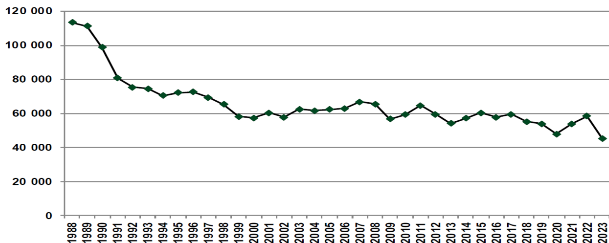
Фигура 2.1.1-10 Общи количества емисии на ПГ без сектор ЗПЗГС за периода 1988-2020 г., Gg CO 2 -екв. (източник UNFCCC)
