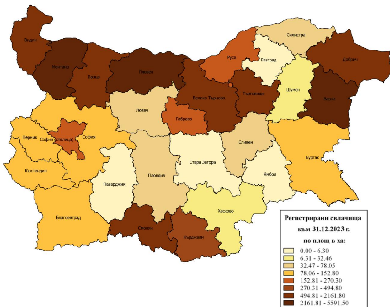
Фигура 2.1.5-4. Разпределение на площите засегнати от свлачищни процеси, ха Източник: ИАОС, Национален доклад за състоянието и опазването на околната среда 2025
