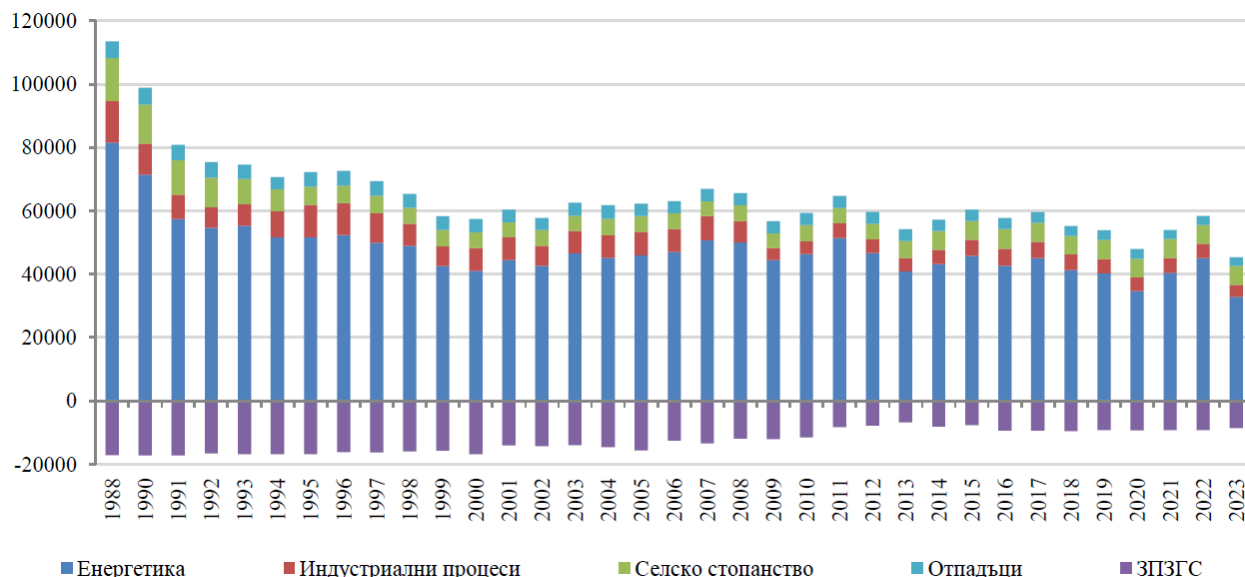
Фигура 2.1.1-13 Общи емисии на парникови газове по сектори за периода 1988-2023 г., Gg CO 2 -екв. (източник UNFCCC)
