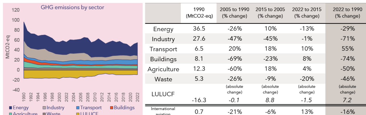
Фигура 2.1.1-12 Изменението на емисиите на ПГ по сектори за периода 1990-2022 г. (източник UNFCCC)
