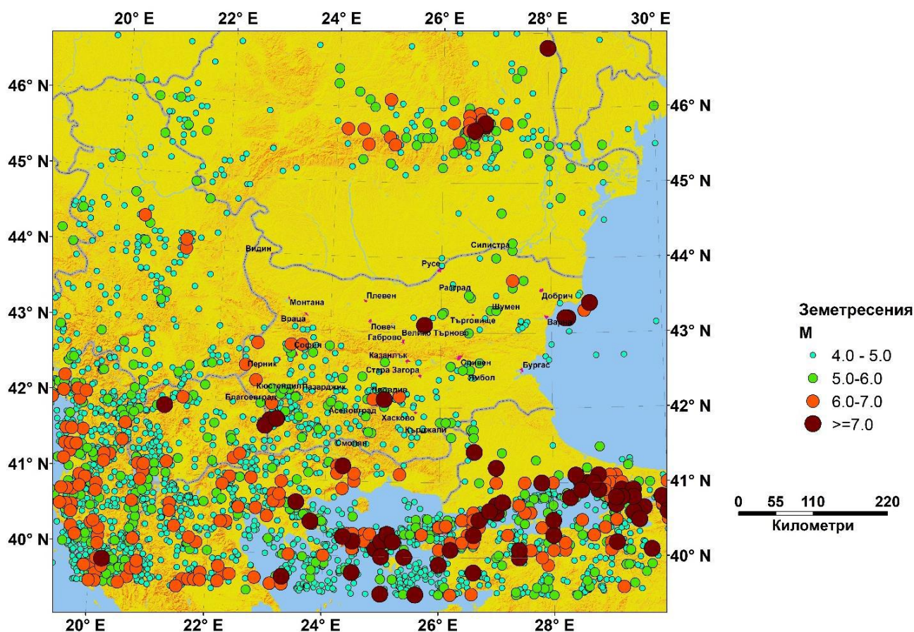
Фигура 2.1.5-5. Пространственото разпределение на земетресенията с магнитуд над 4.0. Източник: НИГГГ-БАН
