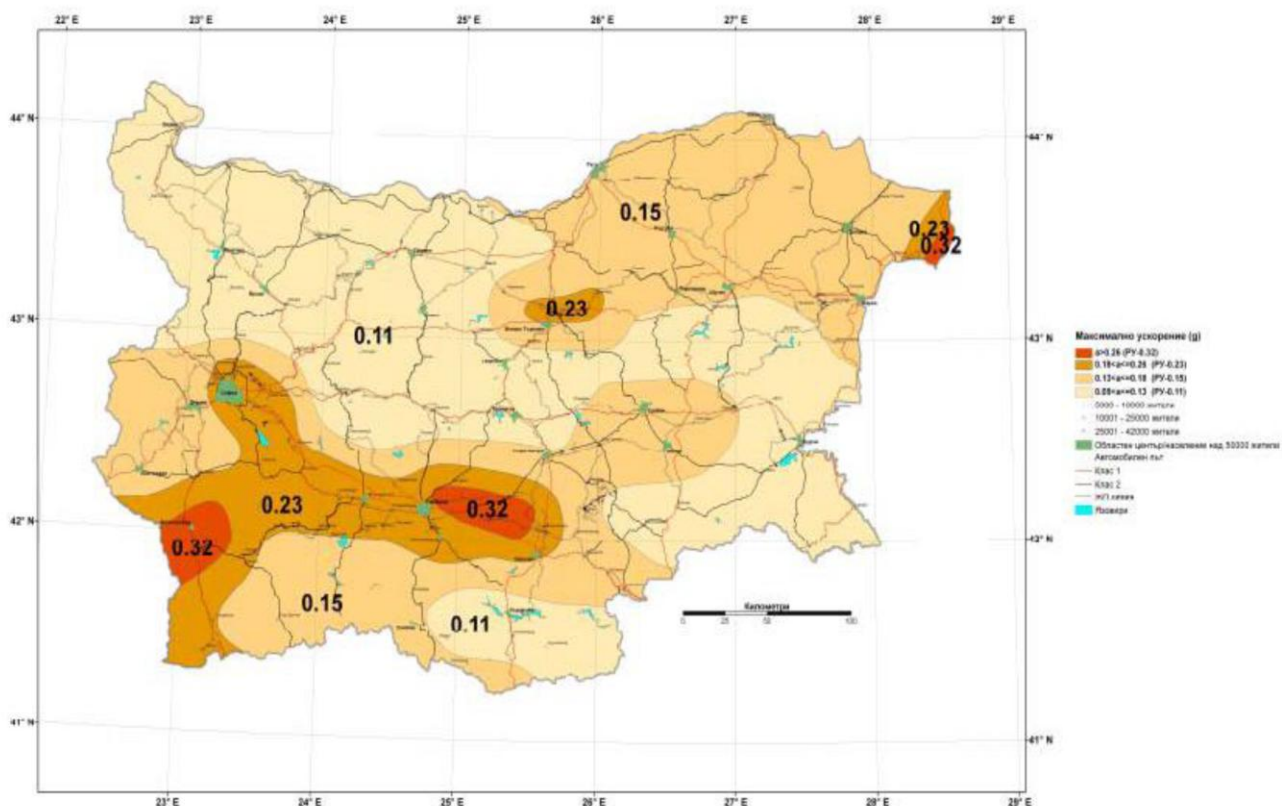
Фигура 2.1.5-7. Карта на максимално ускорение (475г. Период на повторяемост).
