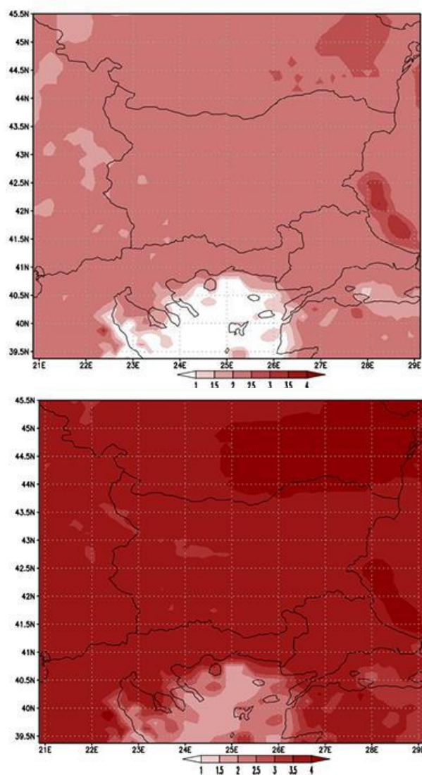
Фигура 2.1.1-8. Тенденция на средногодишната температура - отклонения в ос от нормата 1961 – 1990 г. (източник НИМХ)
